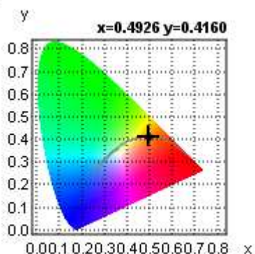
CIE 1931
